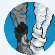
Гидротермальные жерла
